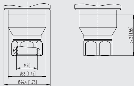
Gewindeanschluss M20
