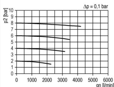
Durchflussdiagramm
