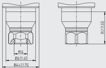
Gewindeanschluss M16
