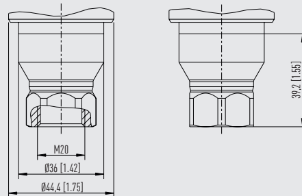
Gewindeanschluss M20
