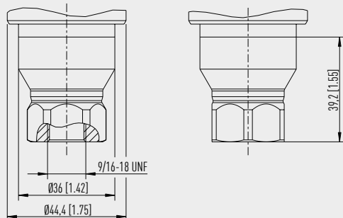
Gewindeanschluss 9/16 - 18 UNF
