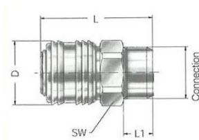
Außengewinde
