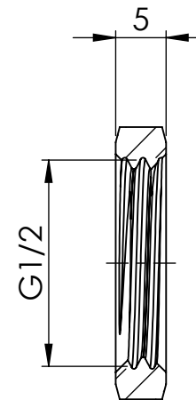
SCHNITT A-A
