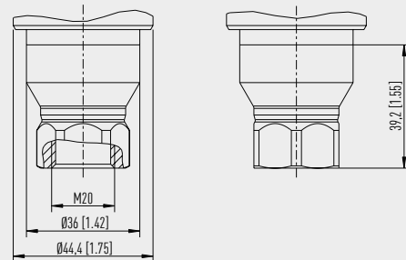
Gewindeanschluss M20
