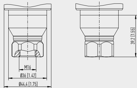
Gewindeanschluss M16
